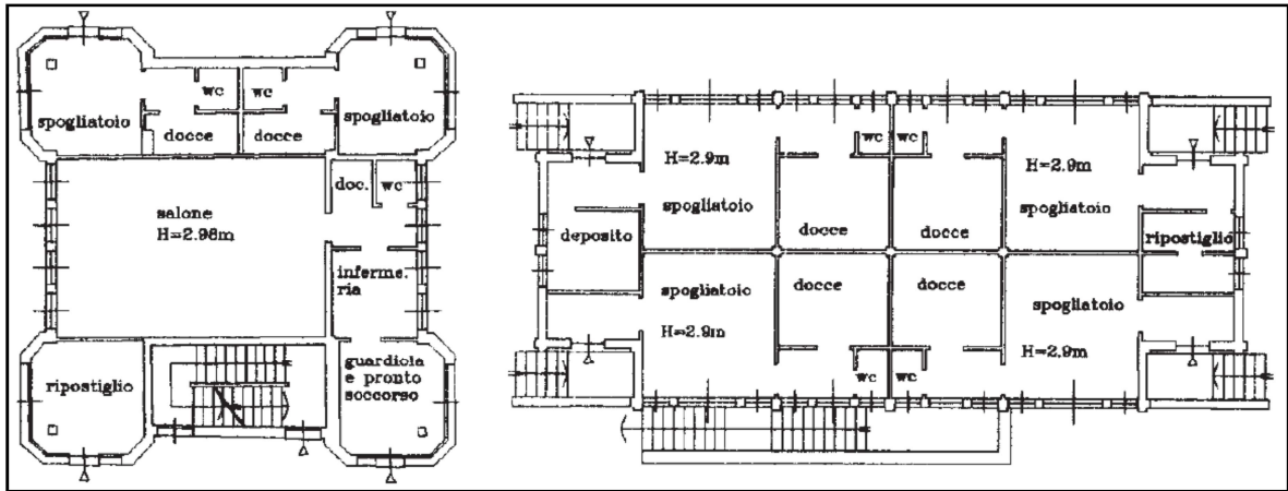
Estratto planimetria Catasto Edilizio Urbano Catasto fabbricati Foglio 1102, Particella 66, Subalterno 2 Fabbricati piano terreno
